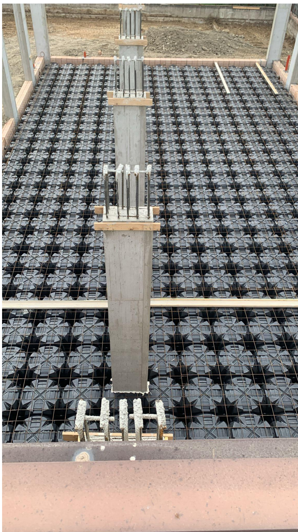
Figura 18 Realizzazione pilastri e platea con vespaio areato, rilievi fotografici del 07/05/2025
