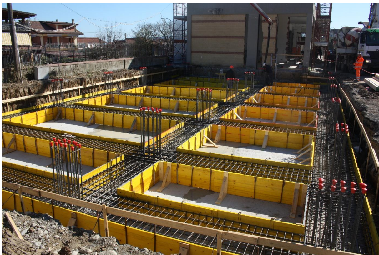
Figura 14 Armatura platea, rilievi fotografici del 20/03/2025
